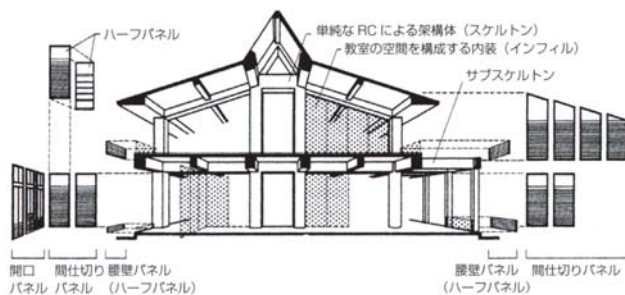
図2 鉄筋コンクリートの構造体と間仕切りパネル
